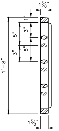
SECTION D-D
