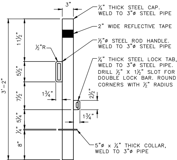
BOLLARD ELEVATION
