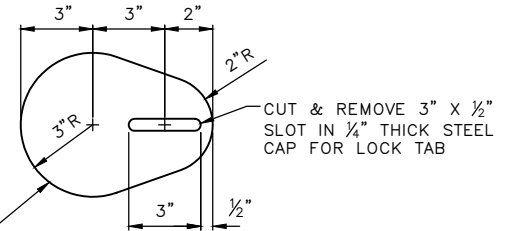
LID - TOP VIEW
