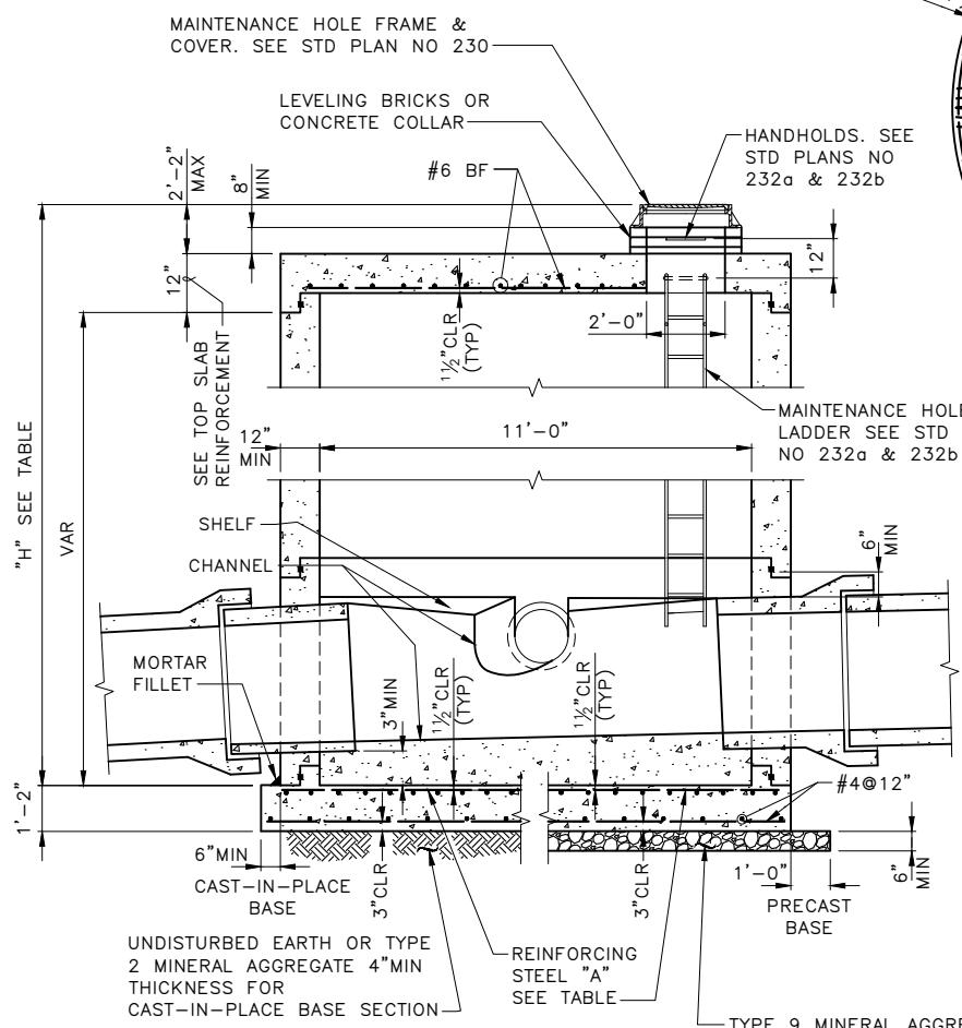
SECTION A-A
